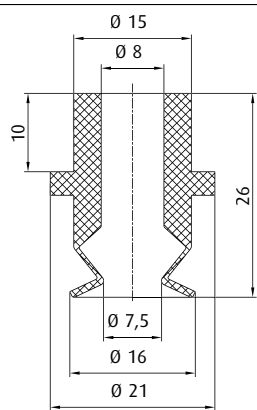
Flachsauger - Serie SL-PF Ø 16 mm
