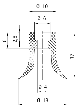
Flachsauger - Serie SL-PF Ø 18A mm
