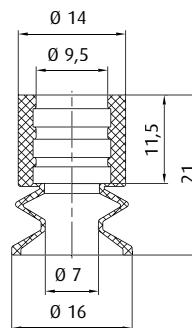
Balgensauger - Serie SL-PB Ø 16 mm
