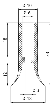
Flachsauger - Serie SL-PF Ø 18 mm
