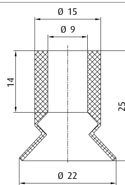
Flachsauger - Serie SL-PF Ø 22 mm
