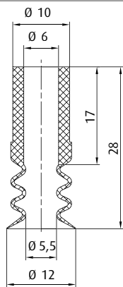
Balgensauger - Serie SL-PB Ø 12 mm
