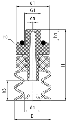
Balgensauger mit Spezialhalter für Saugerplatten - Serie SM-T Ø 18 mm
