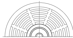
Flachsauger rutschfest mit Innengewinde - Serie SM-PI Ø 20 | 30 | 40 | 50 mm
