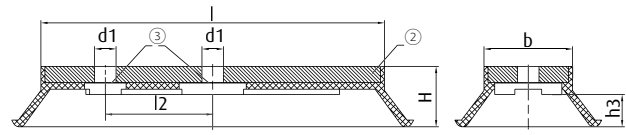
Serie SOPL-A: Material NR orange mit Trägerplatte aus Aluminium
